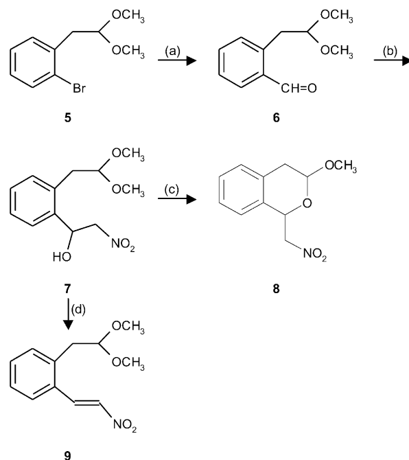
Scheme 1. (a) n -BuLi, THF, -78^\circ\text{C} ; then DMF, ref 14. (b) \text{CH}_3\text{NO}_2 , KOH, \text{CH}_3\text{OH} , \text{H}_2\text{O} , 7 h, 0^\circ\text{C} , 79%. (c) p -TolSO 3 H, \text{CH}_3\text{OH} , 16 h, rt, 40%. (d) \text{CH}_3\text{SO}_2\text{Cl} , \text{NEt}_3 , \text{CH}_2\text{Cl}_2 , 8 h, 0^\circ\text{C} , 79%.
